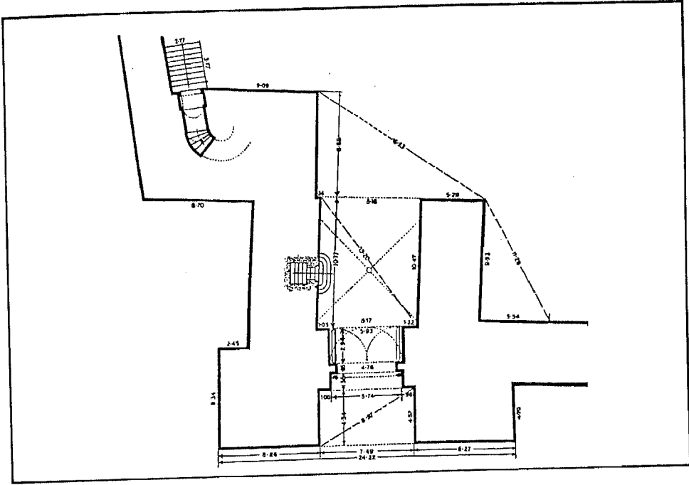
شكل (١١) باب النصر، مسقط عن كزيويل
